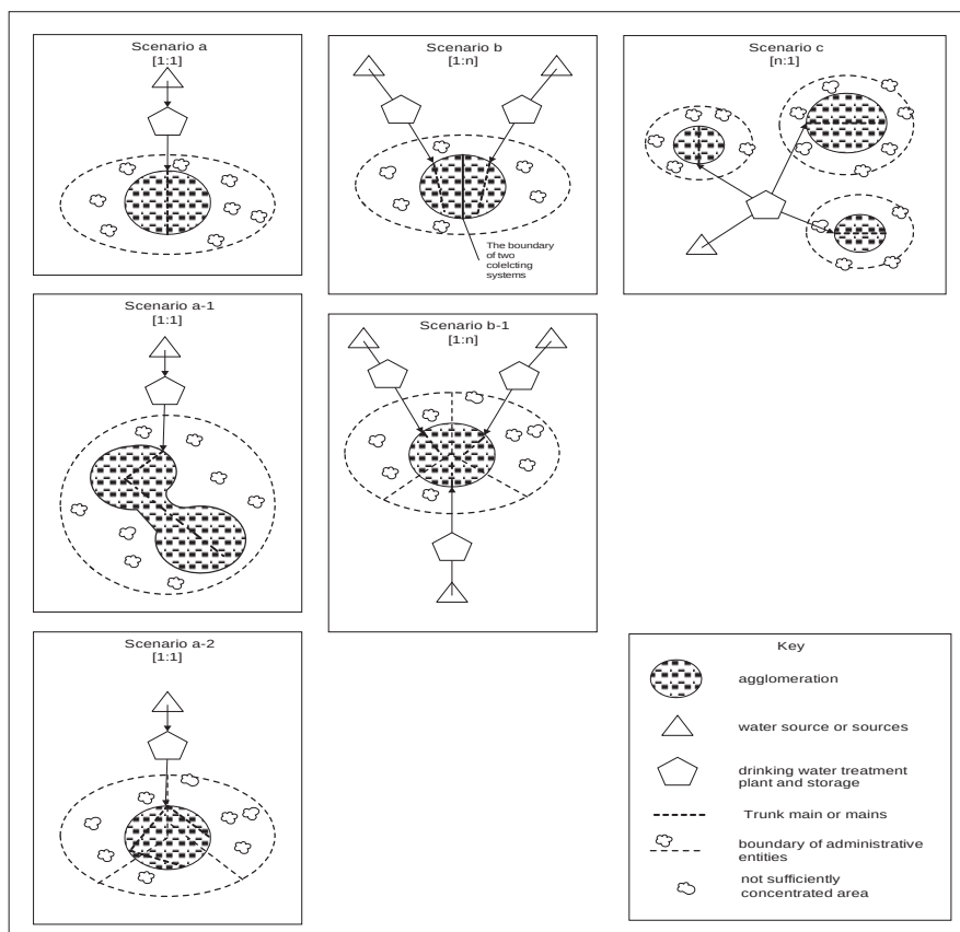
Figura 5.2-2 - Relatii posibile intre aglomerari si statiile de tratare a apei
