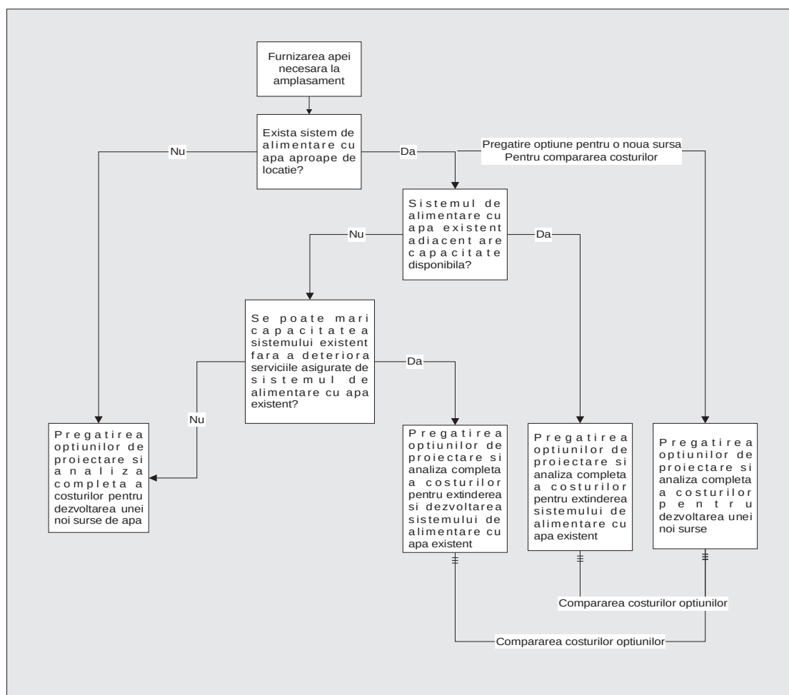
Figura 5.2.-3 - Arborele decizional pentru un nou sistem de alimentare cu apa
