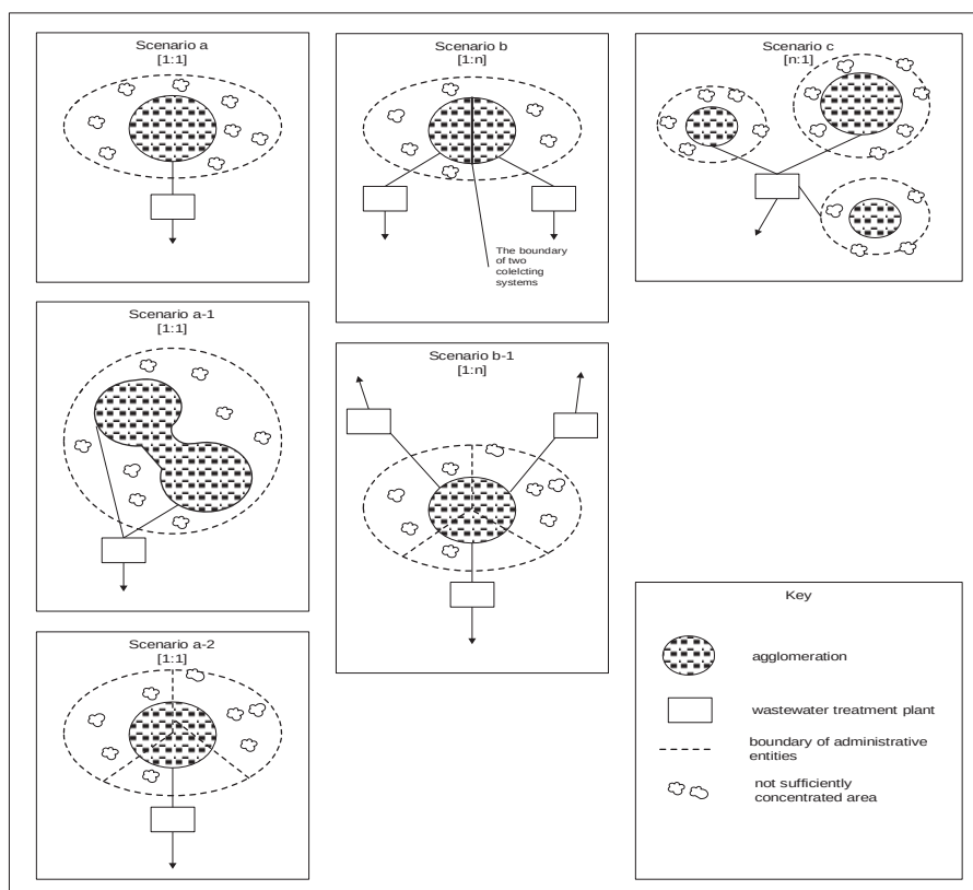
Figura 5.2-1 - Relatii posibile intre aglomerari si statiile de epurare urbane
