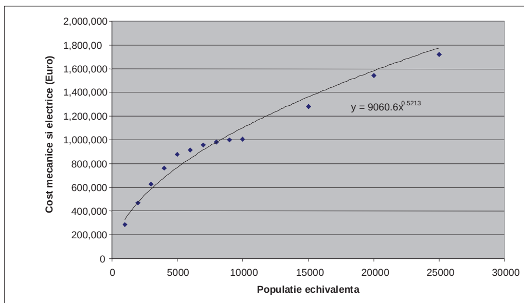
Figura 7.5-3 - Costurile de reabilitare mecanică și electrică
