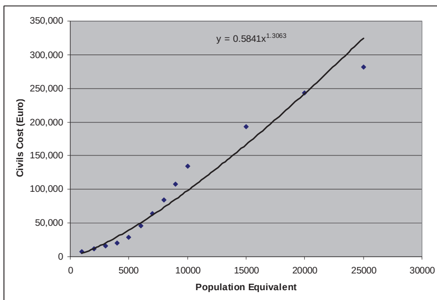
Figura 7.5-4 - Costurile de reabilitare inginerie civila
