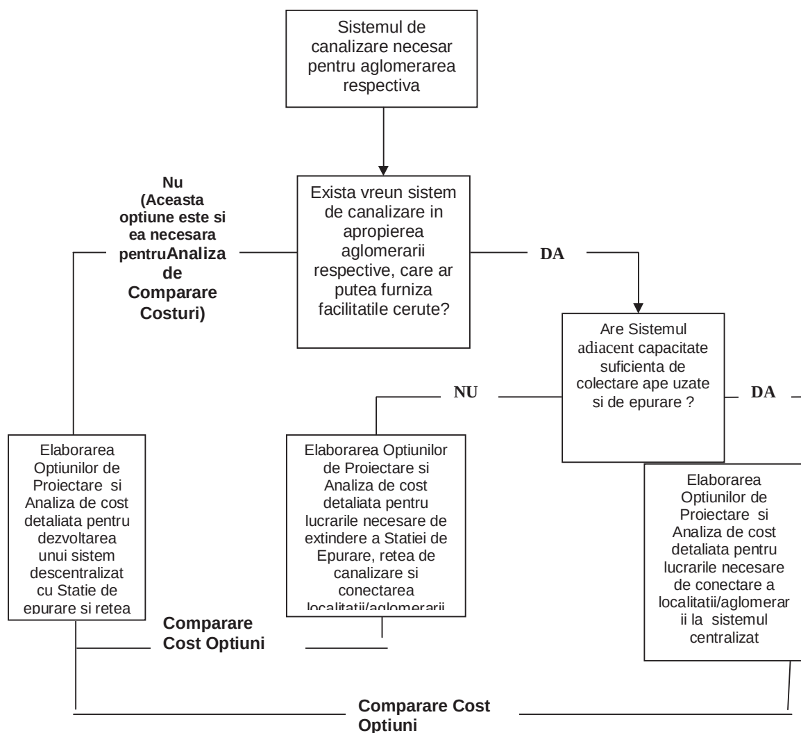
Figura 5.2-4 - Arborele decizional pentru sistemele noi de apă uzată
