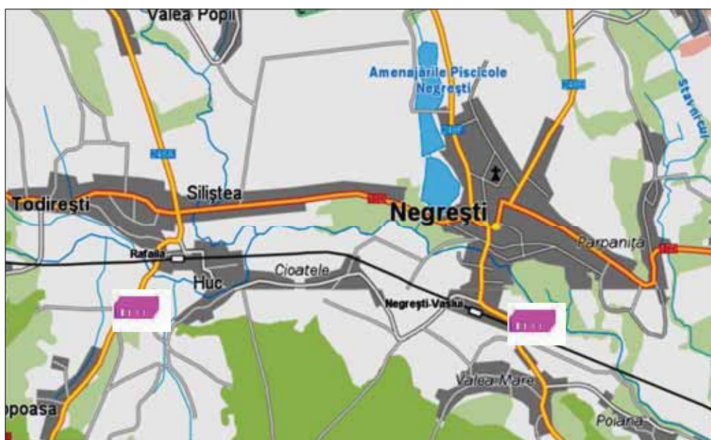
Figura 5.4-6 - Aglomerarea Negresti - colectarea/epurarea apelor uzate: Optiunea 1
