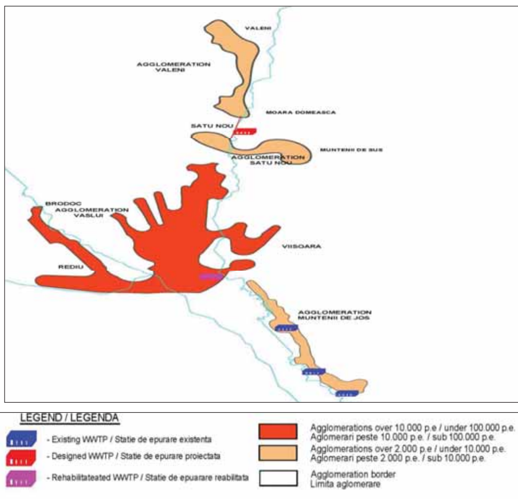
Figura 5.4-2 – Aglomerarea Vaslui- colectarea/epurarea apelor uzate: Optiunea 1
