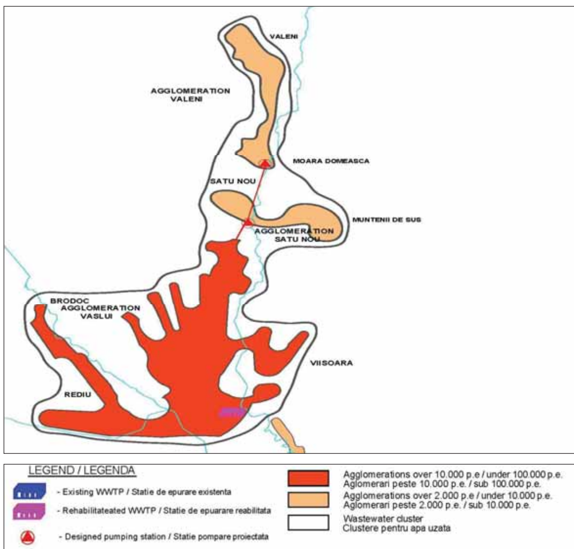
Figura 5.4-3 - Aglomerarea Vaslui- - colectarea/epurarea apelor uzate: Optiunea 2
