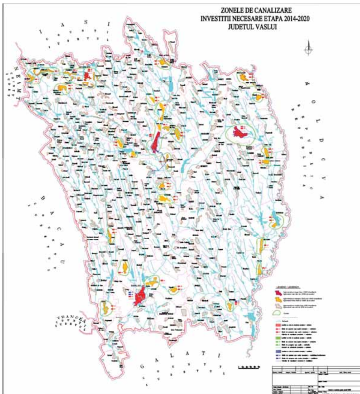
Figura 5.4-1 -Configuratia aglomerarilor > 2000 l.e. din judetul Vaslui
