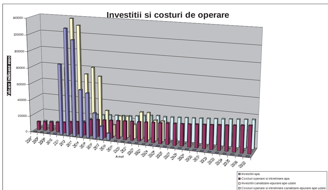
Figura 6.1-2: Costuri de investitii si operare
