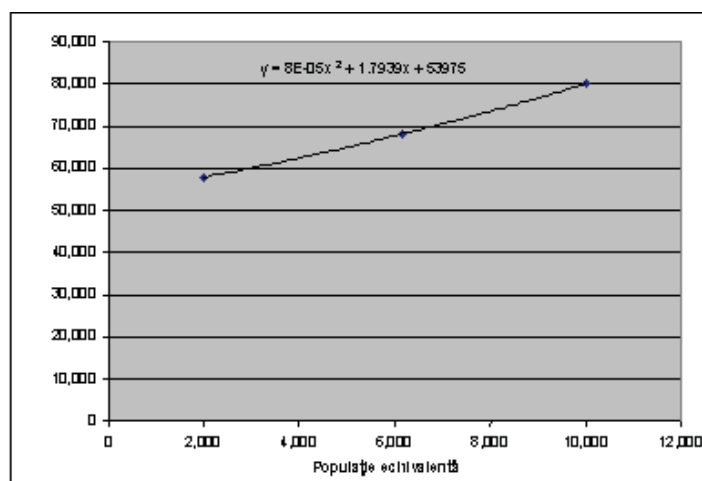
Figura 7.5-6 - Graficul populației echivalente raportată la costul anual de intretinere pentru una SE 1.000p.e. până la 10.000 p.e.
