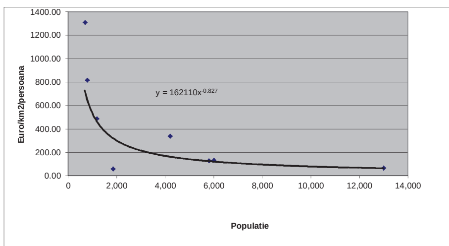
Figura 7.5-1 - Graficul populatiei pe baza costului/km 2 /persoana
